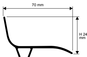
ПЛОСКИЙ ПРОФИЛЬ - АЛЮМ. АНОДИРОВАННЫЙ СЕРЕБРОМ длина бруска 3 Лин.М - упаковка 20шт. - 60 Лин.М
